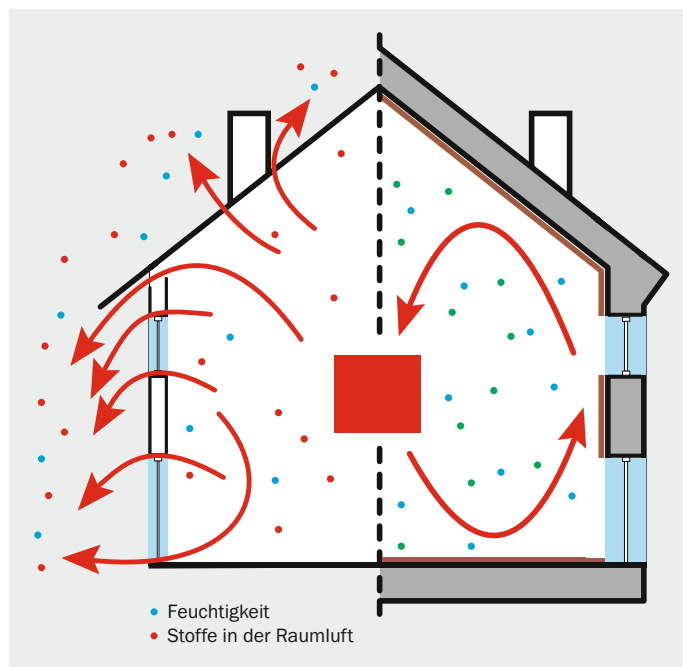
Bauweise früher (links) und heute (rechts) im Vergleich
